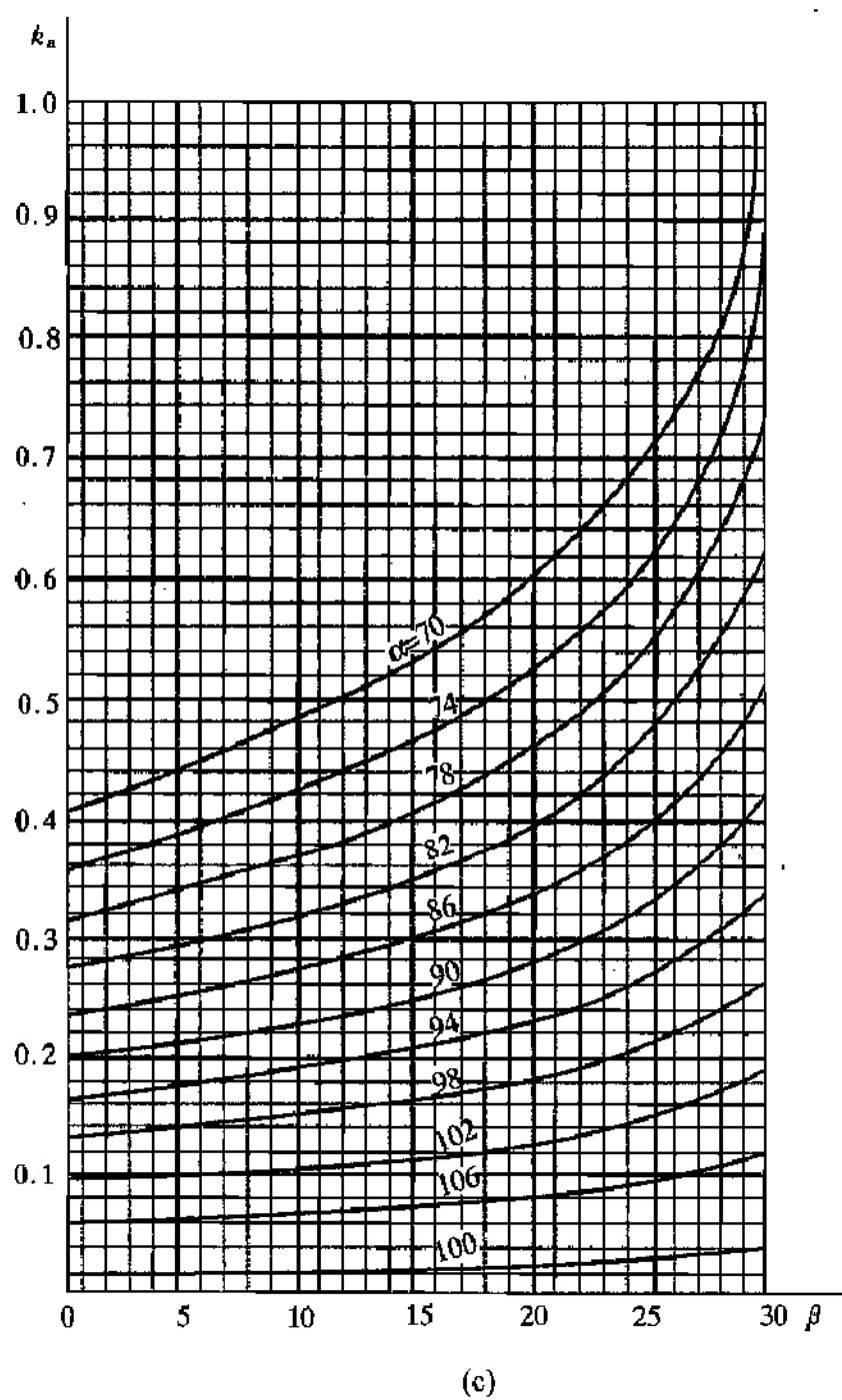
图 L.0.2-3 挡土墙主动土压力系数 k_a (三)
