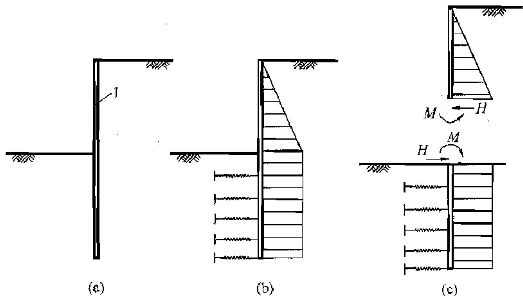
图 55 侧向弹性地基抗力法 1—支护桩
