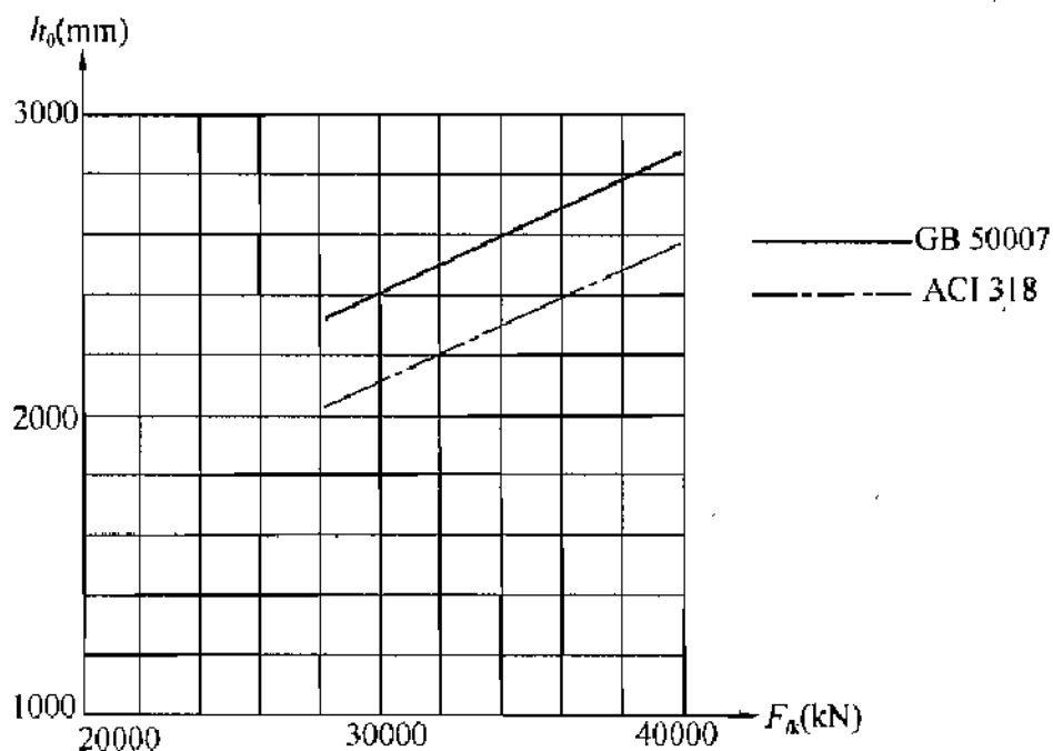
图 50 内柱对承台冲切承台有效高度比较
