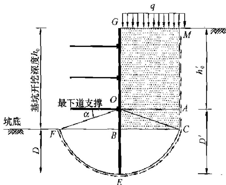
图 56 坑底抗隆起计算简图
