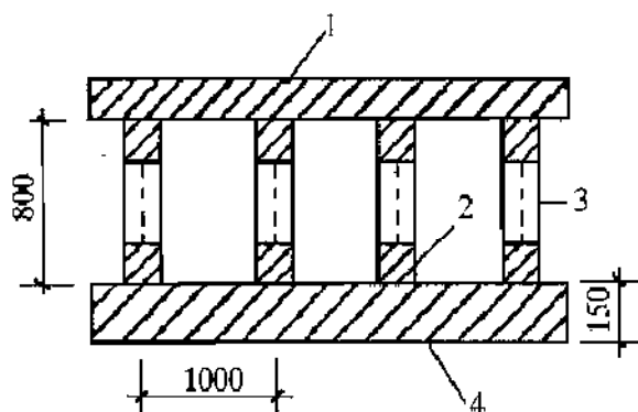
图 39 模型试验加载梁平面图
