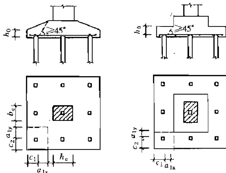
图 8.5.19-2 矩形承台角桩冲切验算
