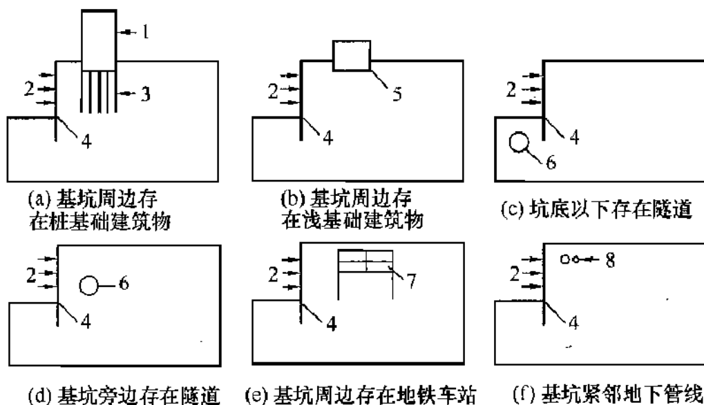
图 53 基坑周边典型的环境条件
