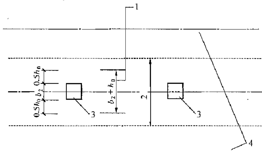
图 43 柱两侧有效宽度范围的示意
