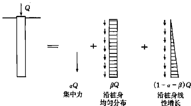
图 R. 0. 4 单桩荷载分担
