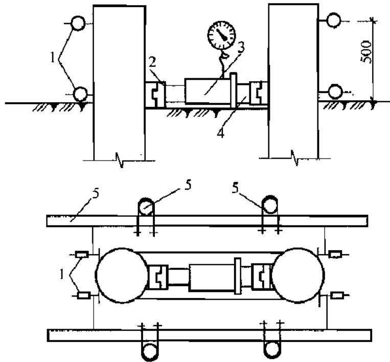
图 S.0.3 单桩水平静载荷试验示意
