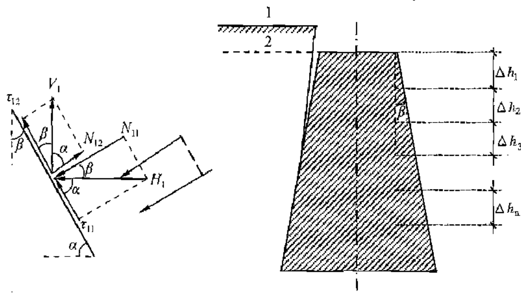
图1 斜面基础基侧受力分布图
