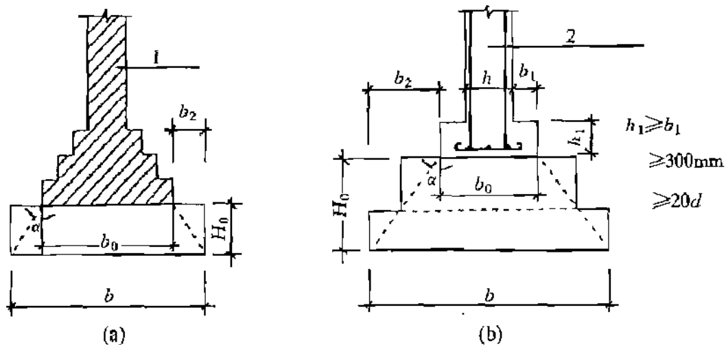
图 8.1.1 无筋扩展基础构造示意
