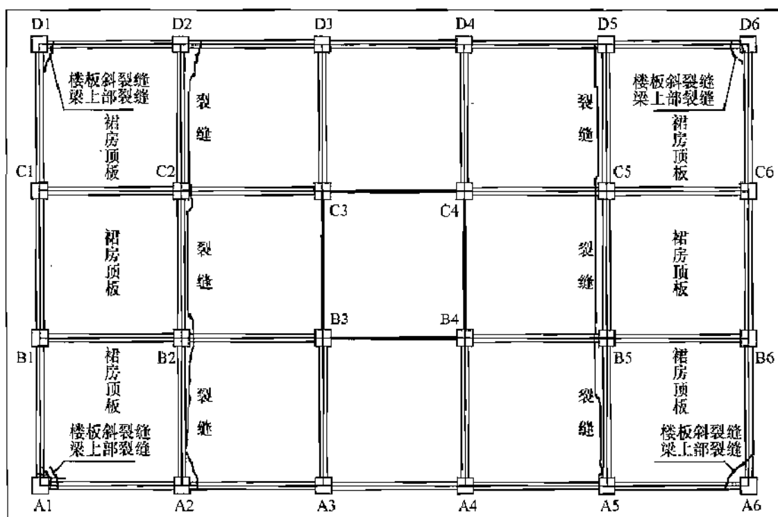
图 48 二层楼板板面裂缝位置图
