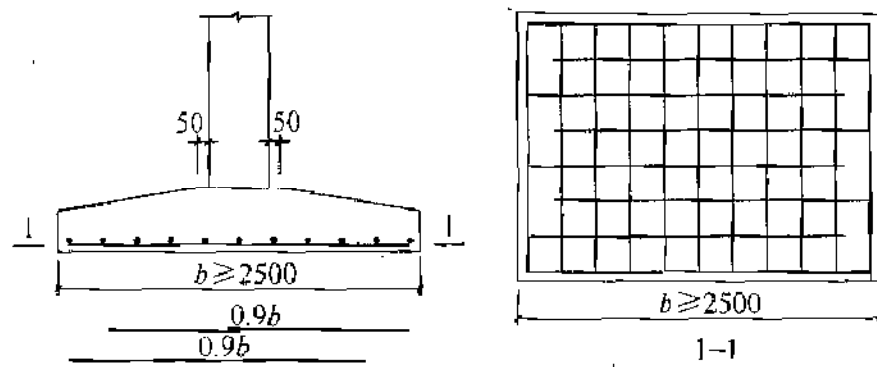
图 8.2.1-1 柱下独立基础底板受力钢筋布置
