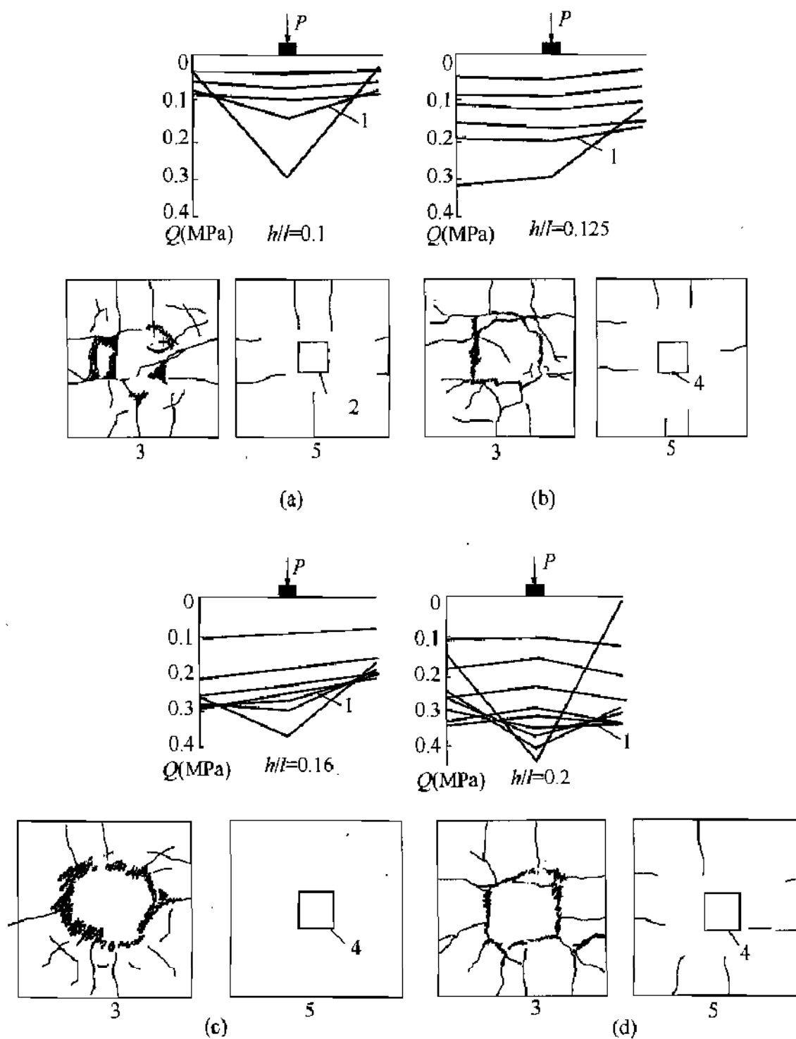
图 31 不同宽高比的基础板下反力分布
