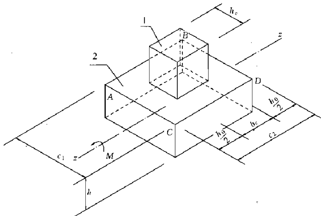
图 8.4.7 内柱冲切临界截面示意
