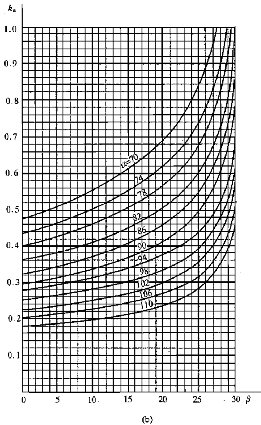
图 L 0.2-2 挡土墙主动土压力系数 k_a (二)
