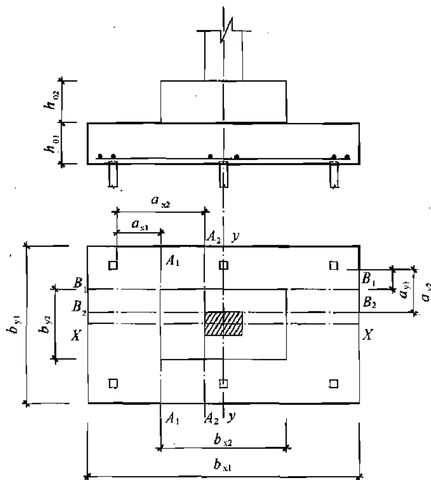
图 U.0.1 阶梯形承台斜截面受剪计算
