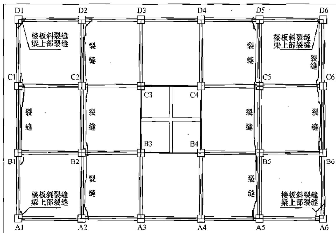
图 47 一层楼板板面裂缝位置图
