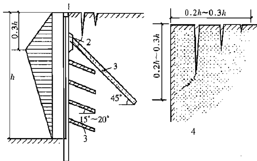
图 25 整体稳定边坡顶部裂隙
