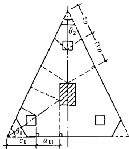
图 8.5.19-3 三角形承台角桩冲切验算
