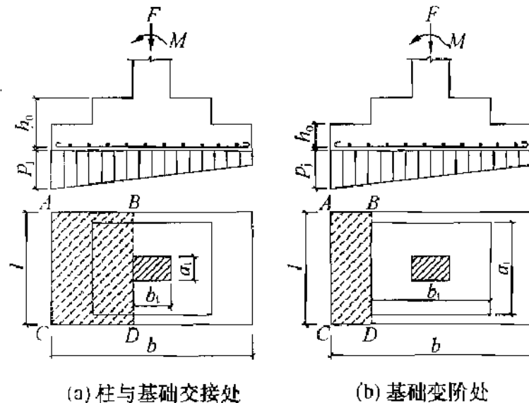
图 8.2.9 验算阶形基础受剪切承载力示意
