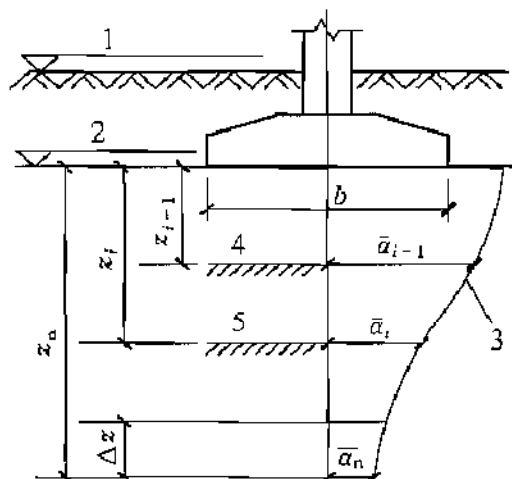
图 5.3.5 基础沉降计算的分层示意
