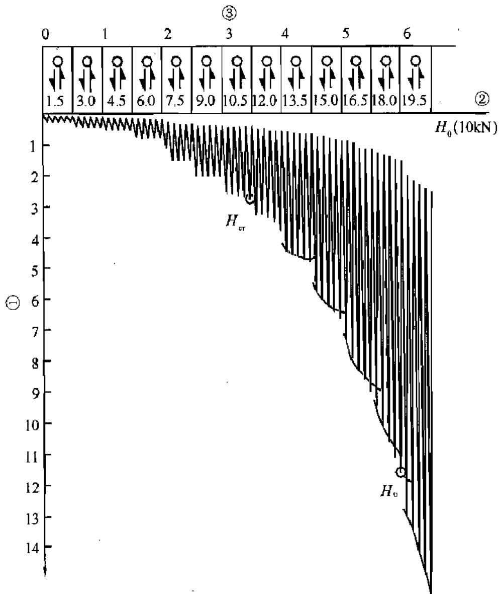
图 S.0.10-1 H_0-t-X_0 曲线
