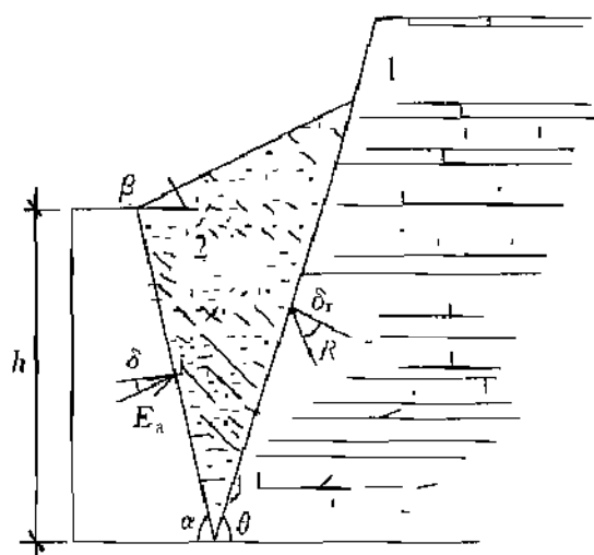
图 6.7.3 有限填土挡土墙土压力计算示意
