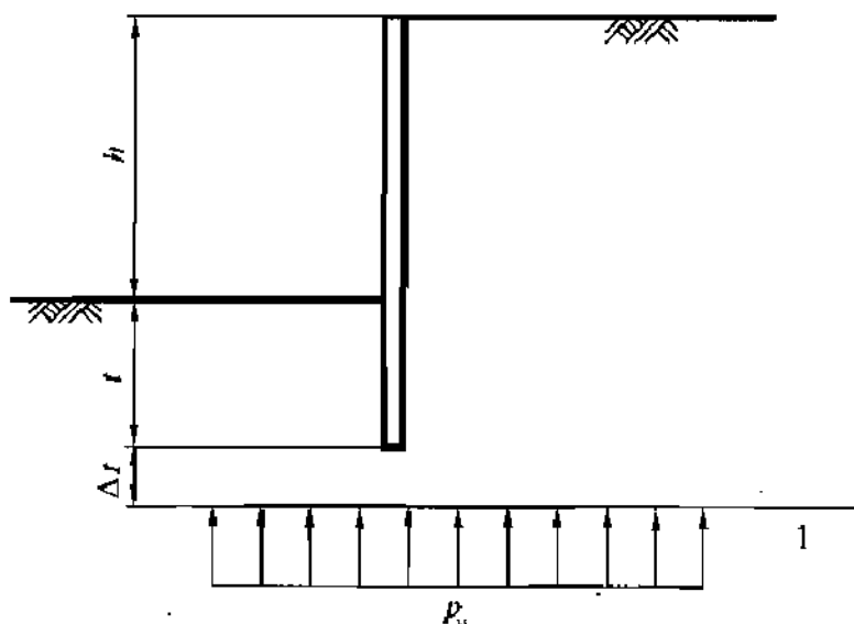
图 W.0.1 基坑底抗渗流稳定验算示意
