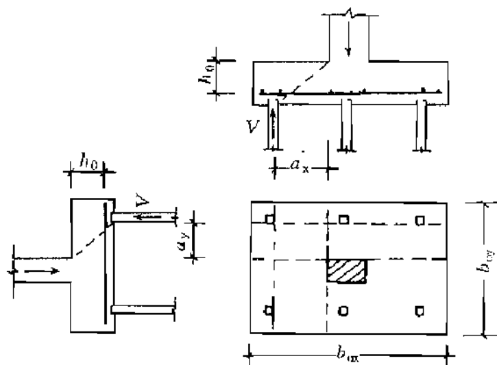
图 8.5.21 承台斜截面受剪计算
