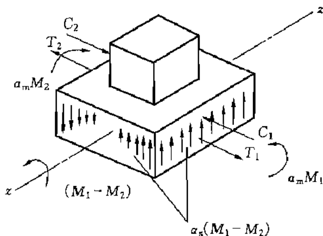
图 32 板与柱不平衡弯矩传递示意
