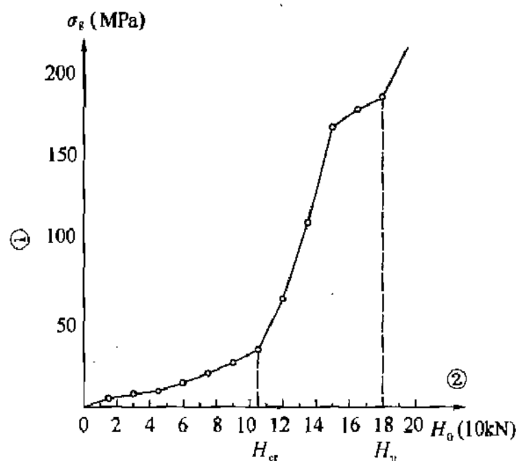
图 S.0.10-3 H_0 - \sigma_g 曲线
