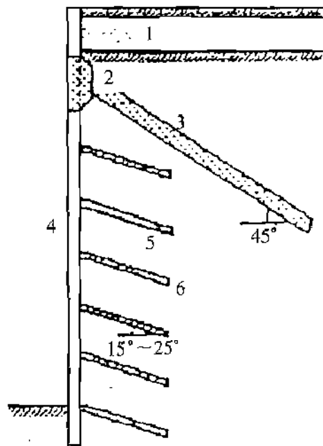
图 6.8.2-2 整体稳定边坡支护
