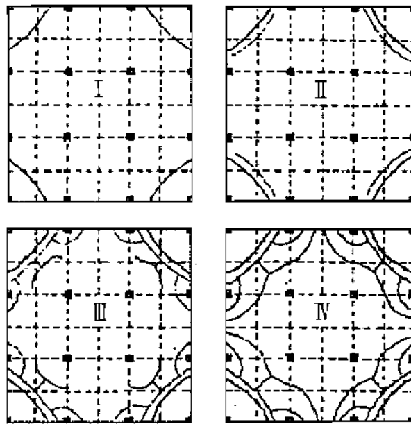
图 37 筏板模型试验裂缝发展过程
