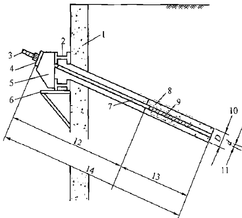
图 59 锚杆构造
