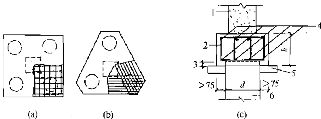
图 8.5.17 承台配筋
