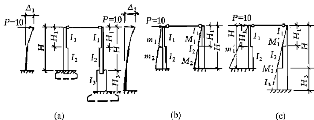
图 29 带短柱基础厂房的计算示意
