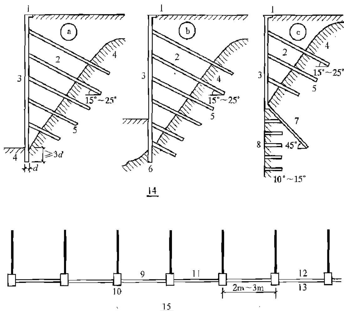
图 6.8.4 锚杆体系支挡结构
