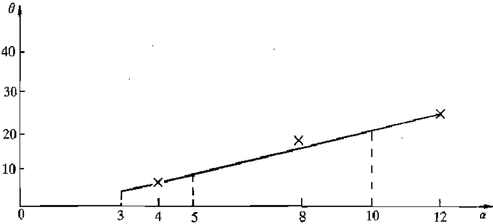
图 9 z=0.25b 时 \alpha-\theta 曲线 (计算值)
