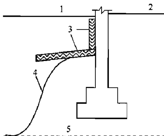
图 4 保温基础示意
