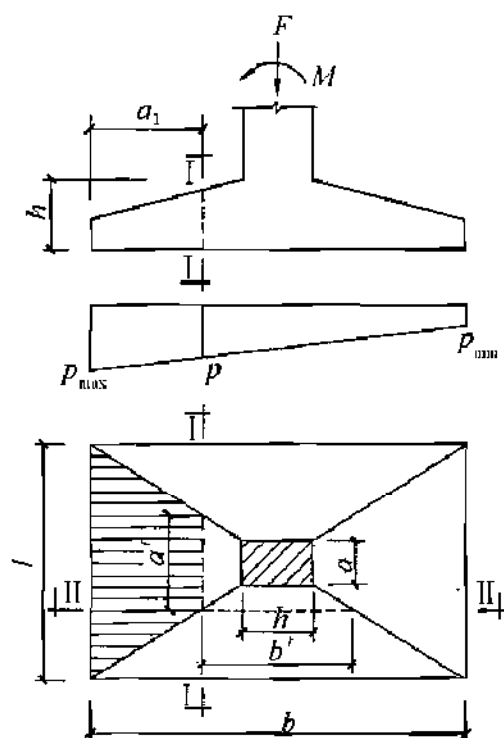
图 8.2.11 矩形基础底板的计算示意
