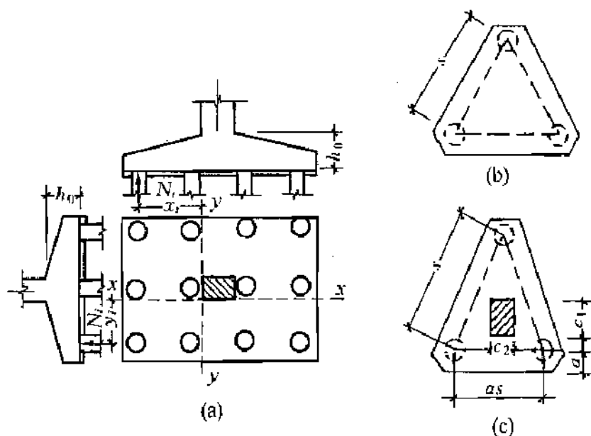
图 8.5.18 承台弯矩计算
