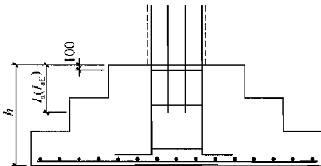
图 8.2.3 现浇柱的基础中插筋构造示意
