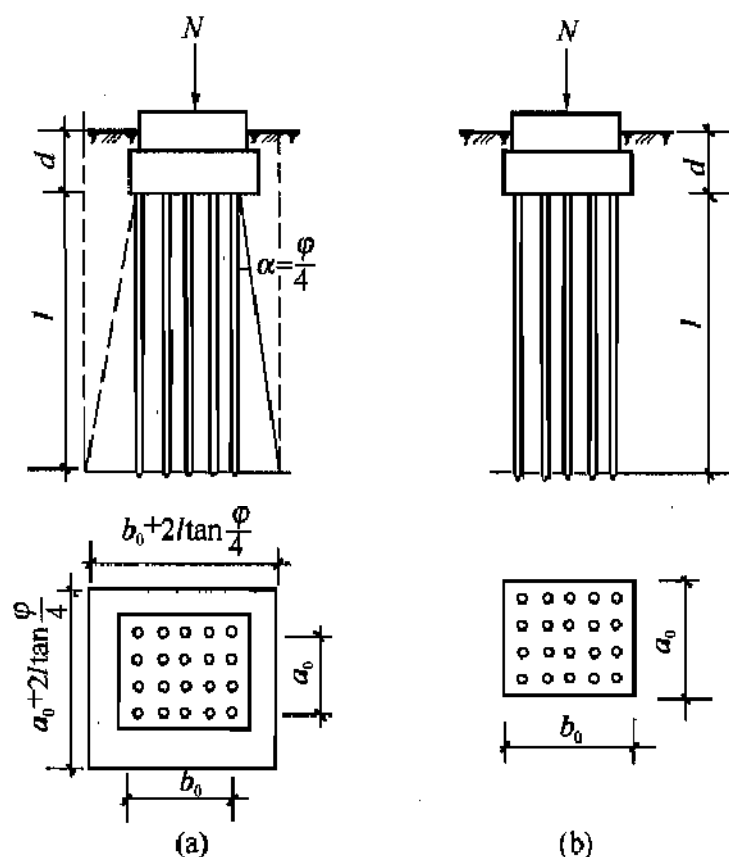
图 R.0.3 实体深基础的底面积
