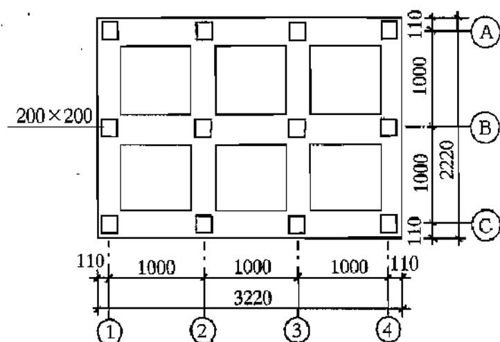
图 39 模型试验加载梁平面图
