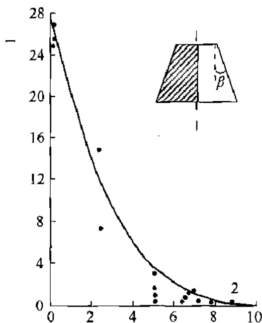
图2 斜面基础的抗冻拔试验
