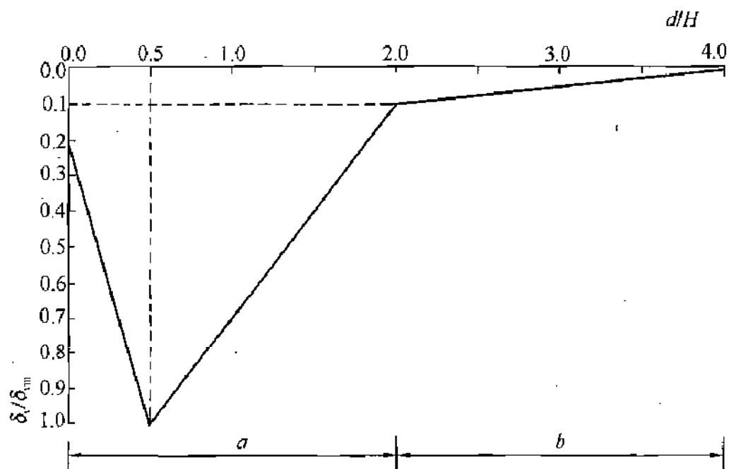
图 54 围护墙后地表沉降预估曲线
