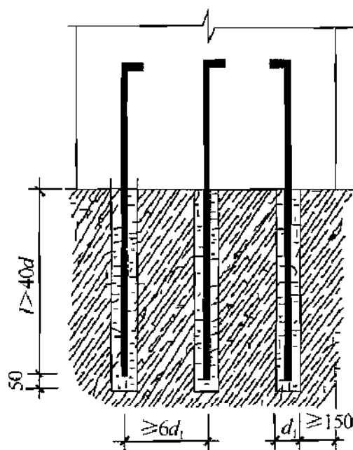
图 8.6.1 锚杆基础
