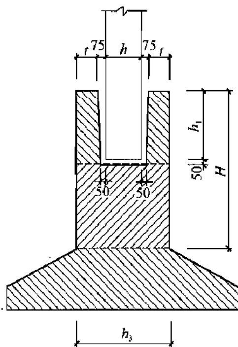
图 8.2.5-1 高杯口基础
