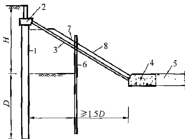
图 57 竖向斜撑体系
