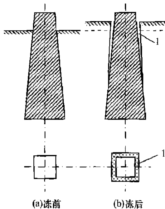
图3 斜面基础的防冻胀试验
