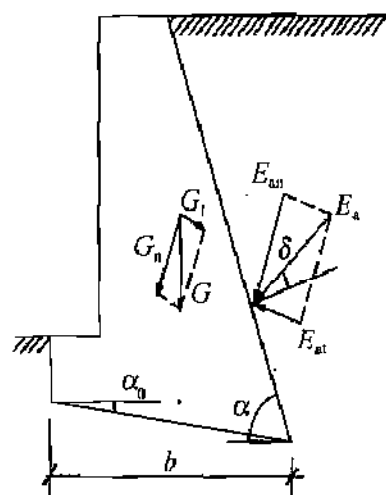
图 6.7.5-1 挡土墙抗滑稳定验算示意
