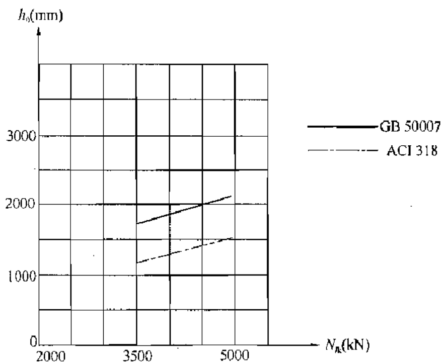
图 51 角桩对承台冲切承台有效高度比较
