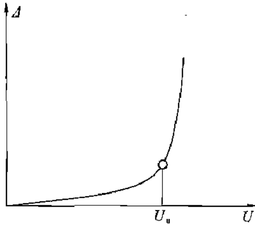
图 T. 0. 10-1 陡变形 U-\Delta 曲线
