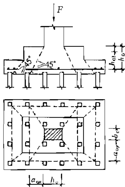
图 8.5.19-1 柱对承台冲切
