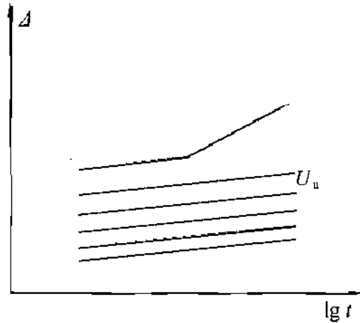
图 T. 0. 10-2 \Delta-\lg t 曲线
