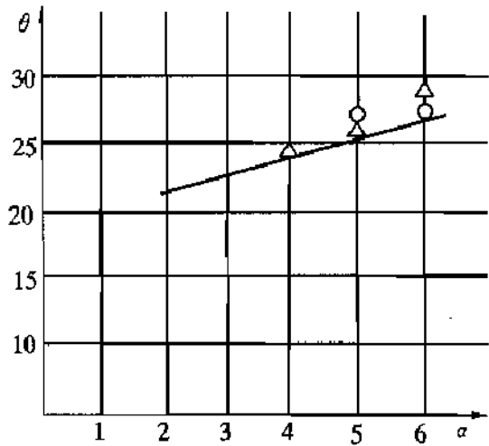
图 7 双层地基试验 \alpha - \theta 曲线 △—室内试验；○—现场试验
