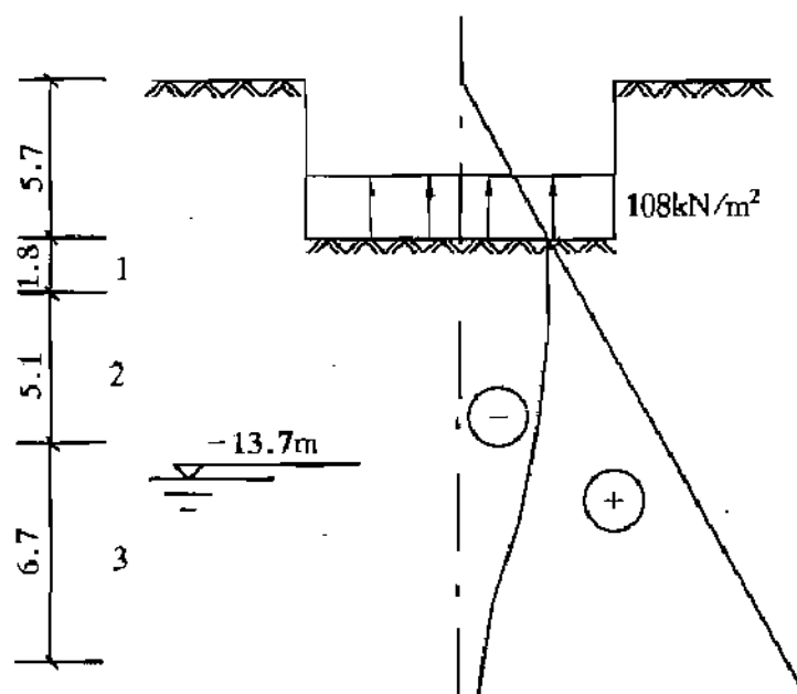
图 11 回弹计算示意
