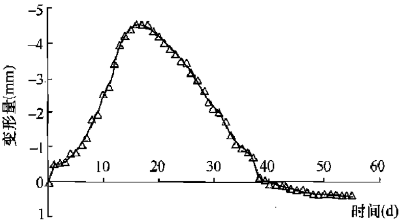
图 17 3 号刚性变形深标点变形时程曲线
