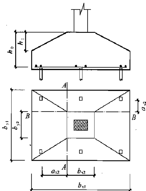
图 U.0.2 锥形承台受剪计算
