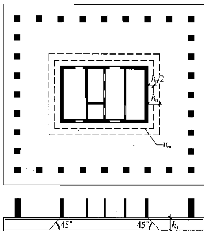
图 8.4.8 筏板受内筒冲切的临界截面位置
