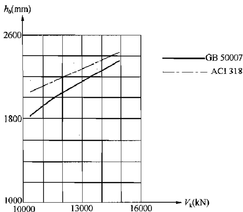
图 52 柱边剪切承台有效高度比较
