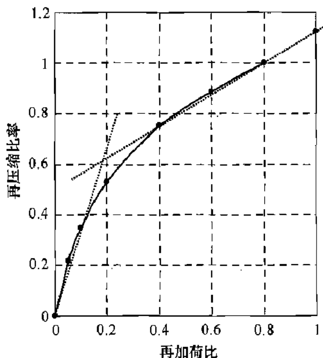
图 15 载荷试验再压缩曲线规律
