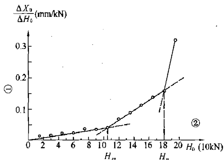
图 S.0.10-2 H_0 - \Delta X_0 / \Delta H_0 曲线
