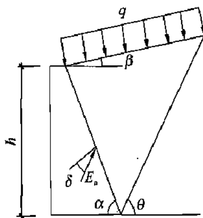
图 L. 0.1 计算简图
