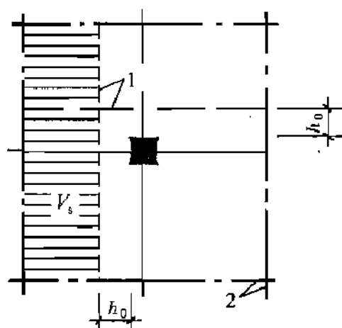
图35 内柱(筒)下筏板验算 剪切部位示意
