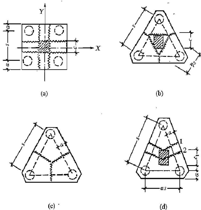
图 49 承台破坏模式
