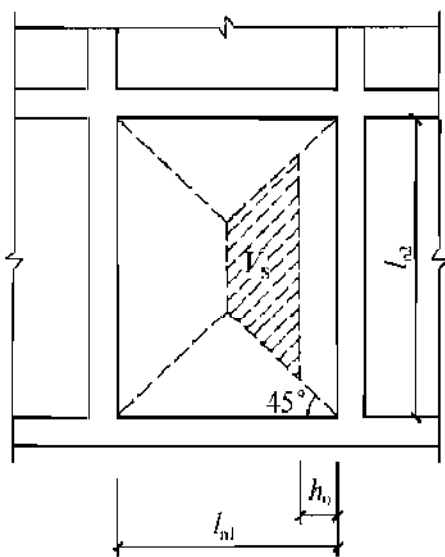
图 8.4.12-2 底板剪切 计算示意
