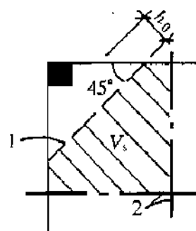
图36 角柱(筒)下筏板验算 剪切部位示意
