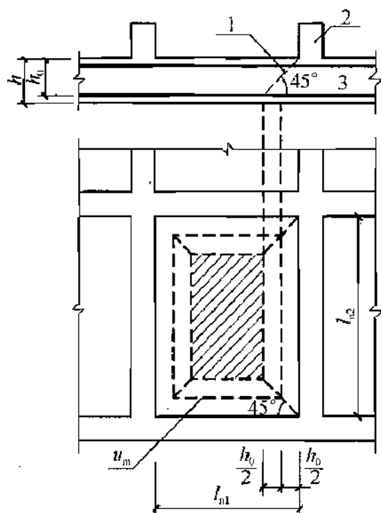
图 8.4.12-1 底板的冲切计算示意
