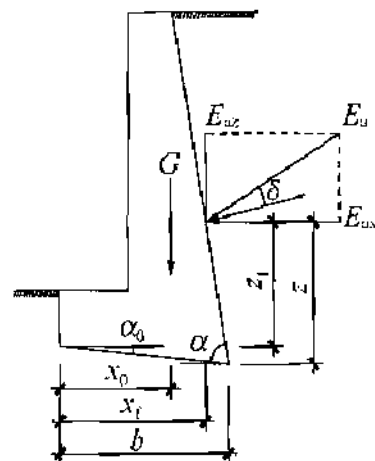
图 6.7.5-2 挡土墙抗倾覆稳定验算示意
