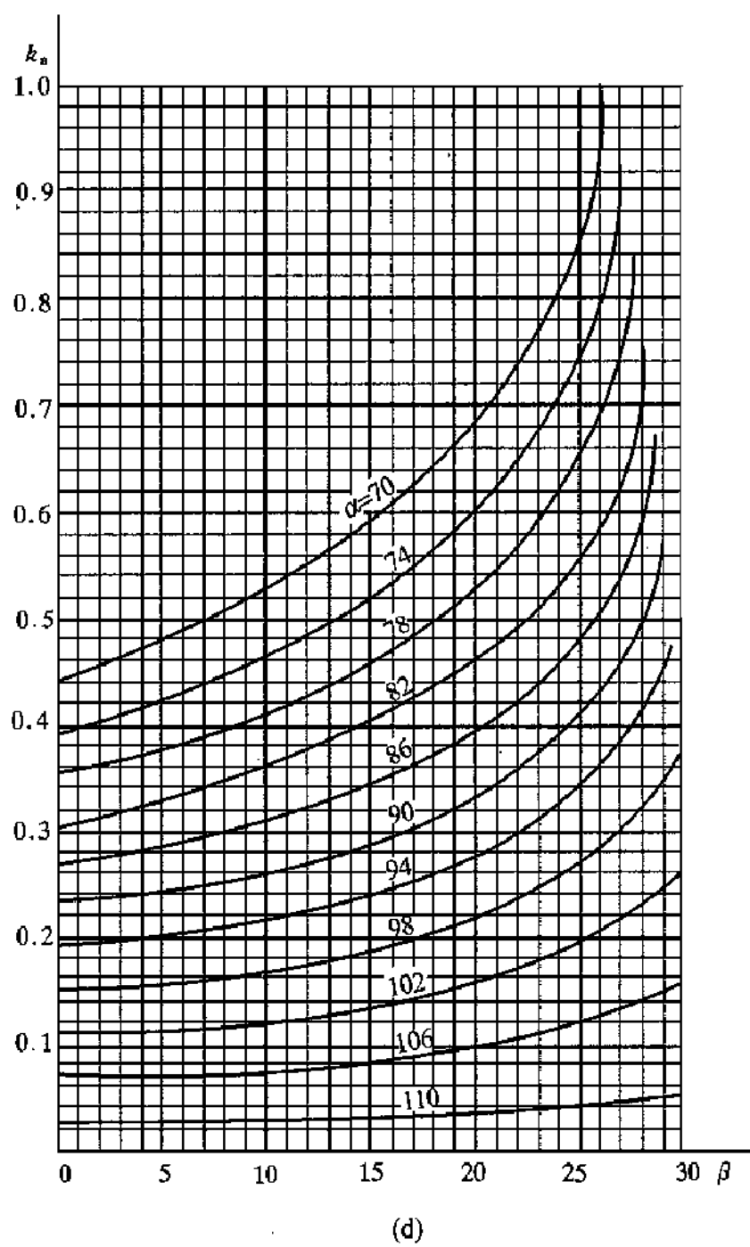
图 L. 0. 2-4 挡土墙主动土压力系数 k_a (四)
