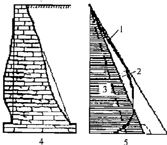
图 24 墙体变形与土压力
