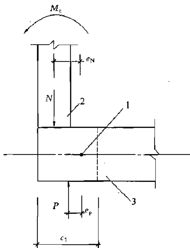
图 33 边柱 M_{\text{unb}} 计算示意
