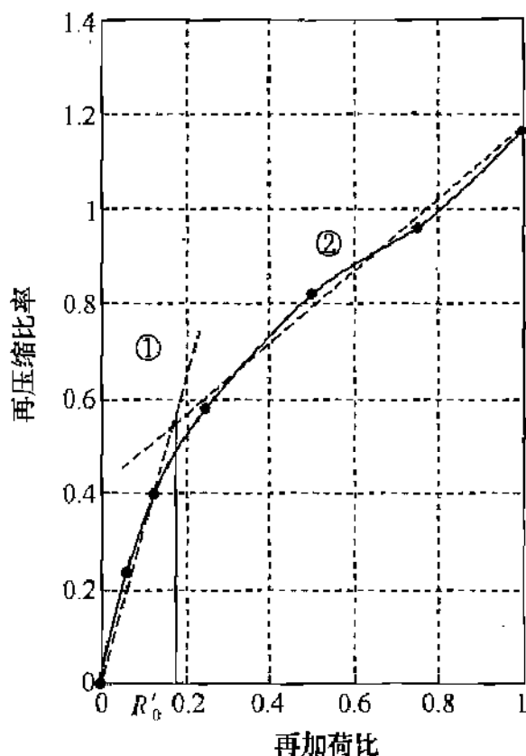
图 12 再压缩比率与再加荷比关系
