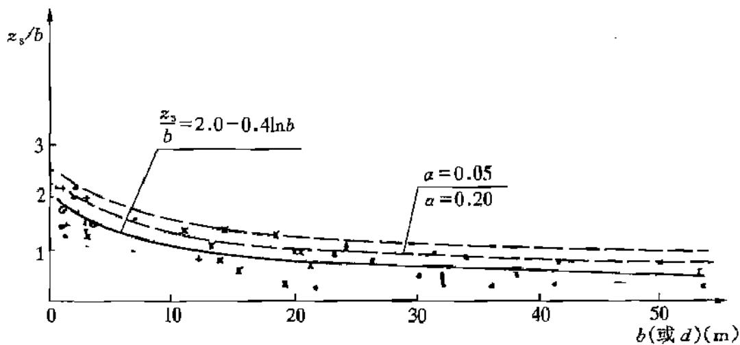
图 10 z_s/b 实测点和回归线
