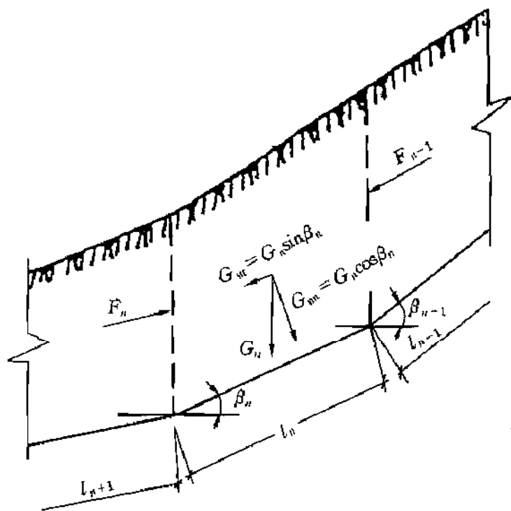
图 6.4.3 滑坡推力计算示意
