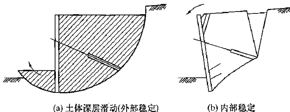
图 58 锚杆的整体稳定
