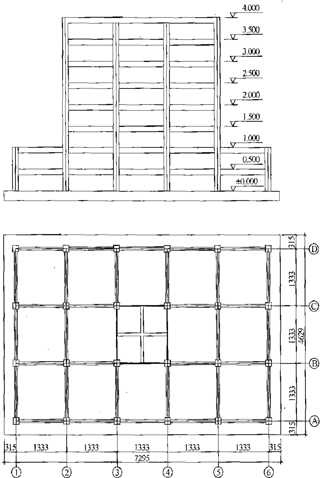
图 46 大底盘结构试验模型平面及剖面
