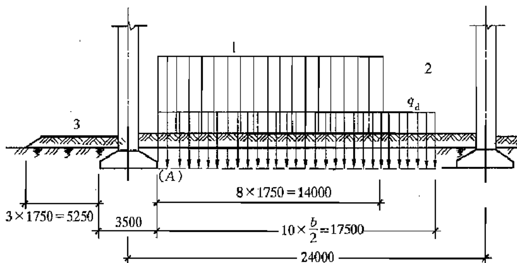
图 28 地面荷载计算示意
