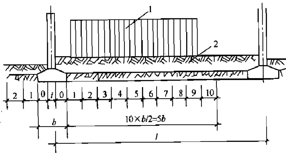
图 N.0.4 地面荷载区段划分
